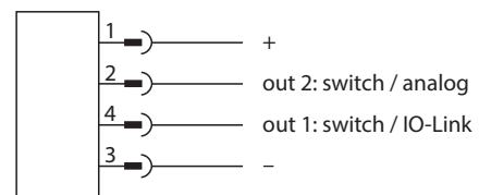
Abb. 15: Anschlussbild TS...2LIUPN...
