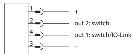
Abb. 17: Anschlussbild TS...2UPN...
