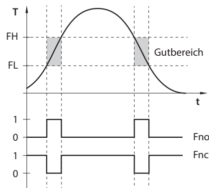
Abb. 7: Verhalten des Schaltausgangs – Fensterfunktion
