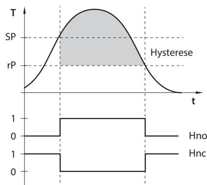
Abb. 8: Verhalten des Schaltausgangs – Hysterese Funktion
