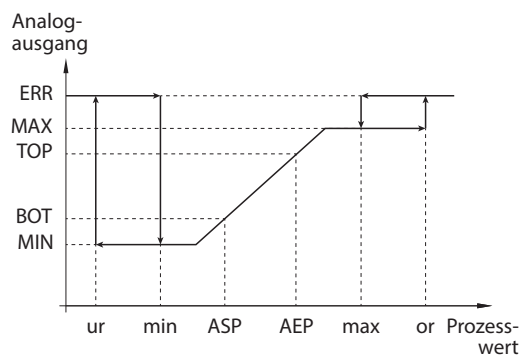
Abb. 9: Steigende Ausgangskennlinie
