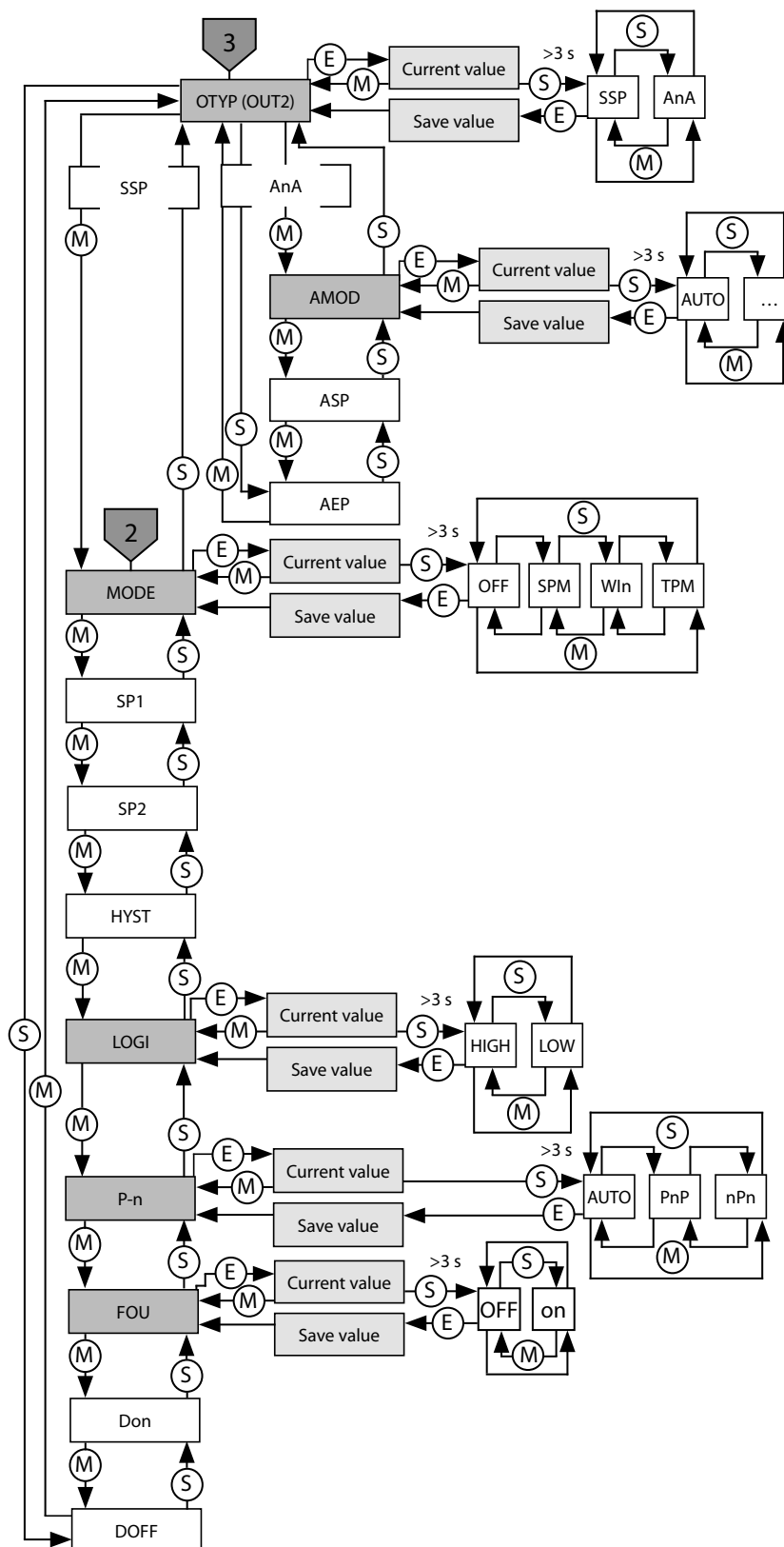
Abb. 21: Untermenü Ausgänge (OUT...)
