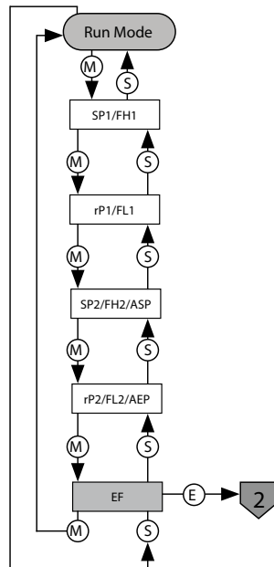
Abb. 26: Hauptmenü in der VDMA-Menüführung
