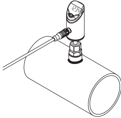
Abb. 12: Montage TS700
