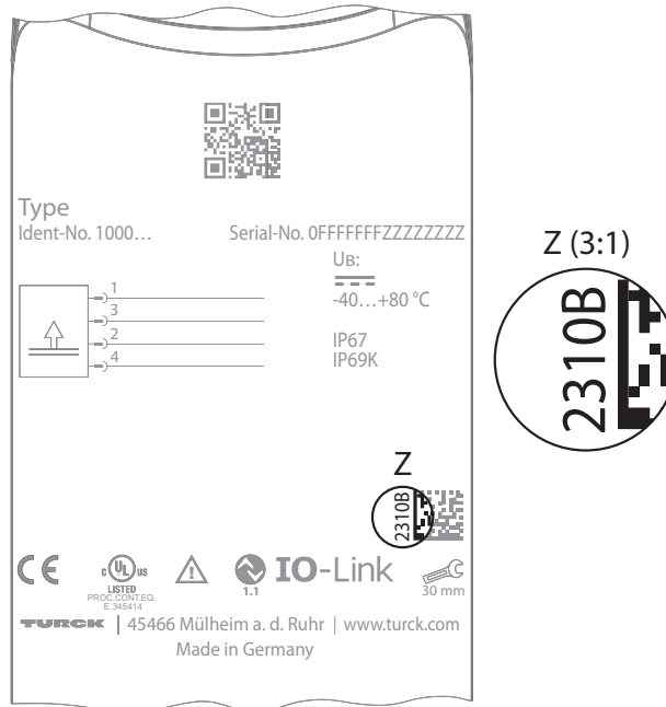
Abb. 1: Produktionsdatum auf Gehäuserückseite
