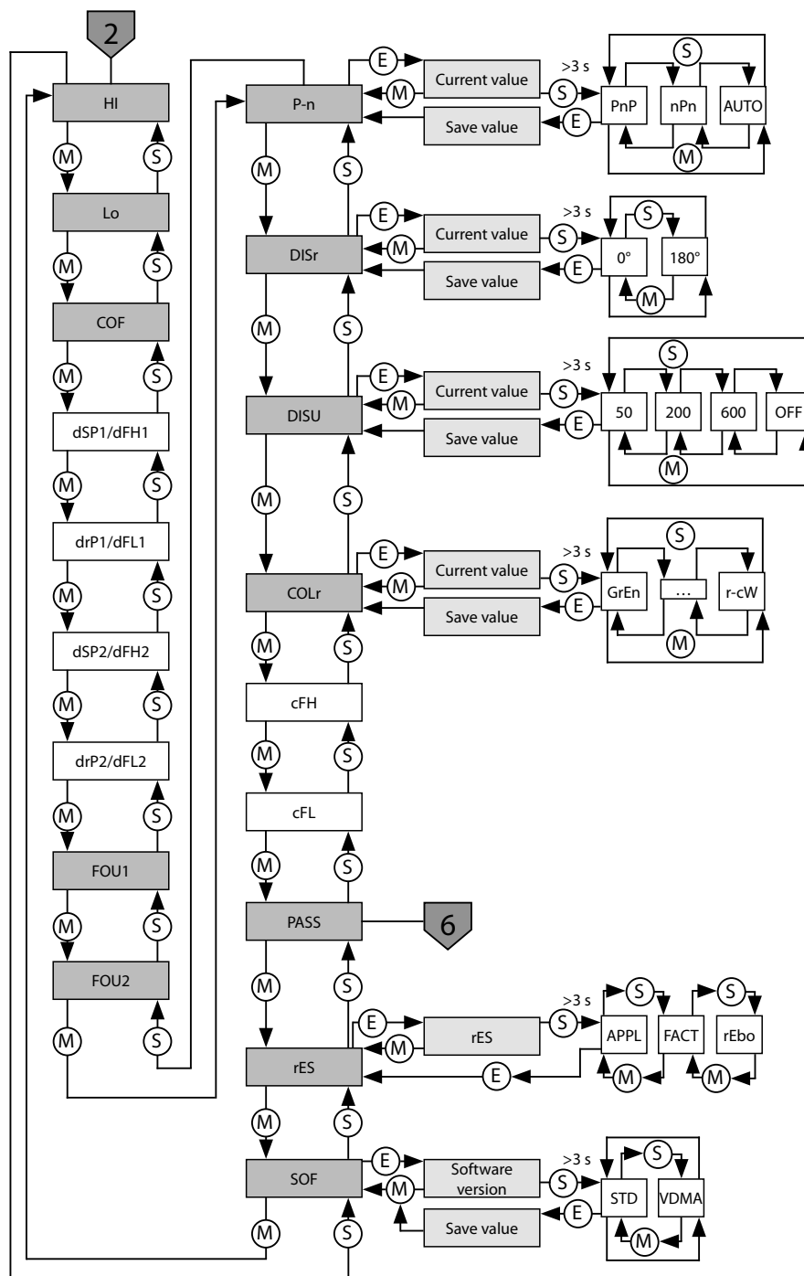
Abb. 25: Untermenü Extended Functions (EF) im Legacy Mode
