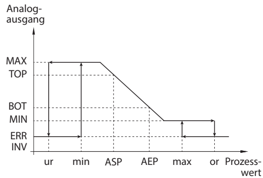
Abb. 10: Fallende Ausgangskennlinie, MIN \neq 0
