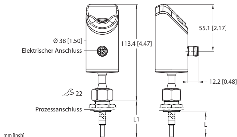
Abb. 13: Elektrischer Anschluss für Steuerung
