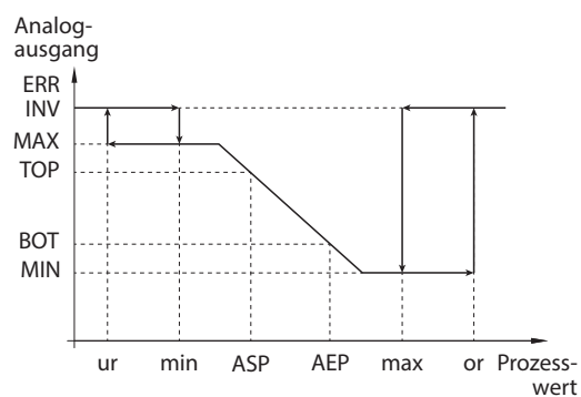
Abb. 11: Fallende Ausgangskennlinie, MIN = 0
