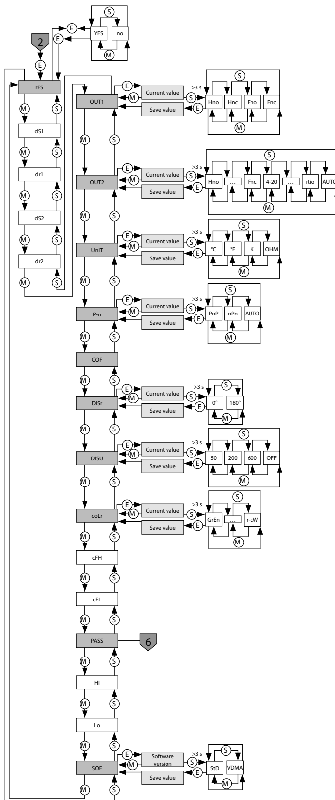
Abb. 27: Untermenü Extended Functions (EF) in der VDMA-Menüführung
